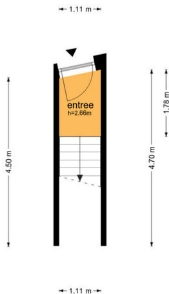
Nieuwe Noord 38 P - Hoorn Eerste Verdieping
