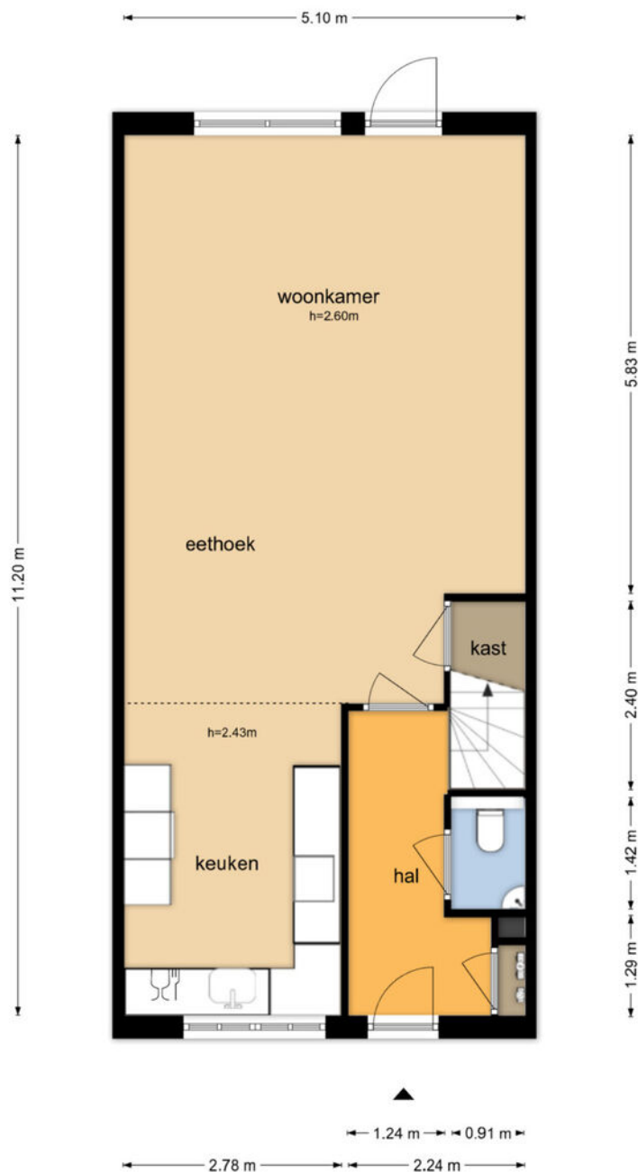
Catshoek 5 - Alkmaar Begane Grond
